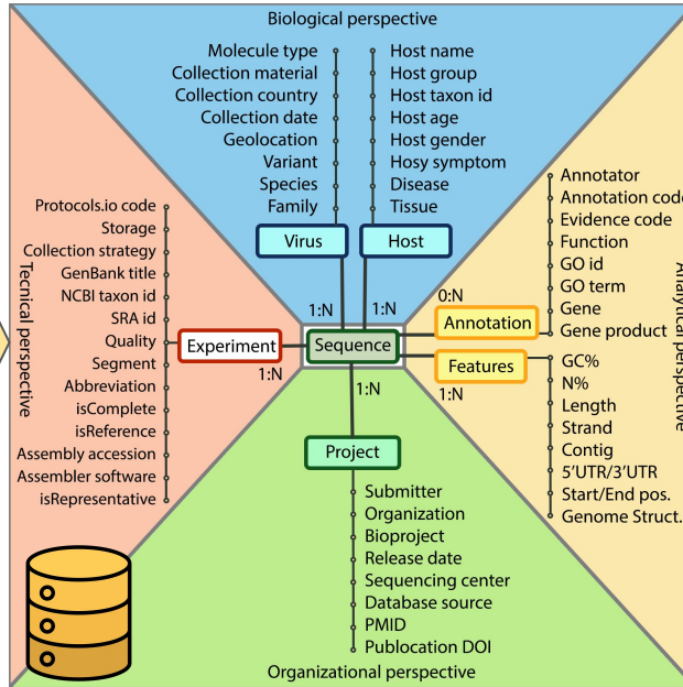
VJDB metadata schema v0.1
